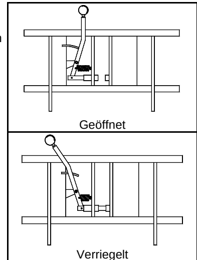
Abb. 2 Verriegeln des Arbeitswerkzeuges
