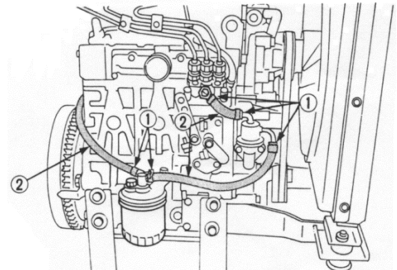
2) Kraftstoffleitungen
