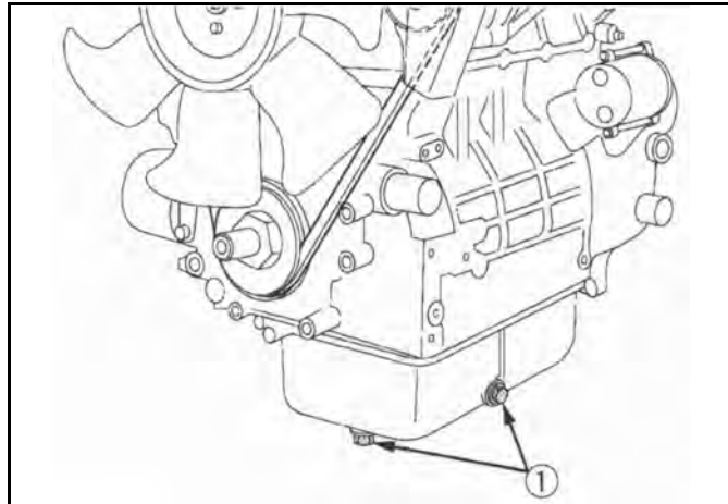
1) Ölablass-Schraube
