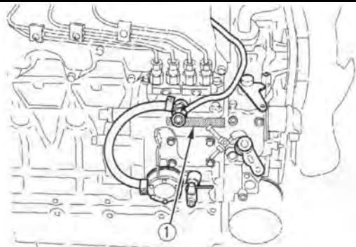
Motornummer eingeschlagen
