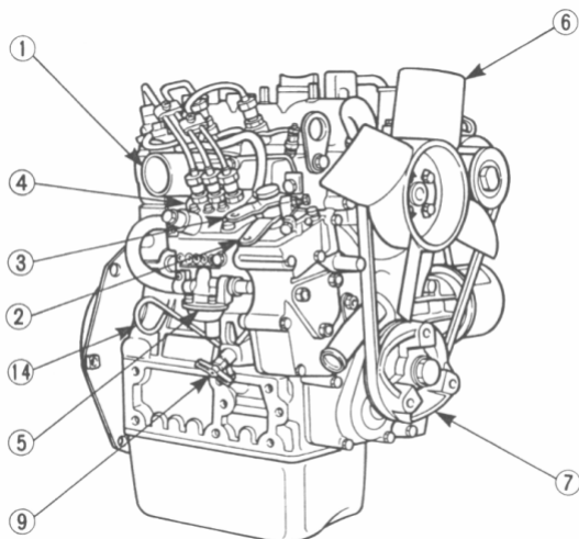
Hoflader 217S/ 221S/ 222S:
