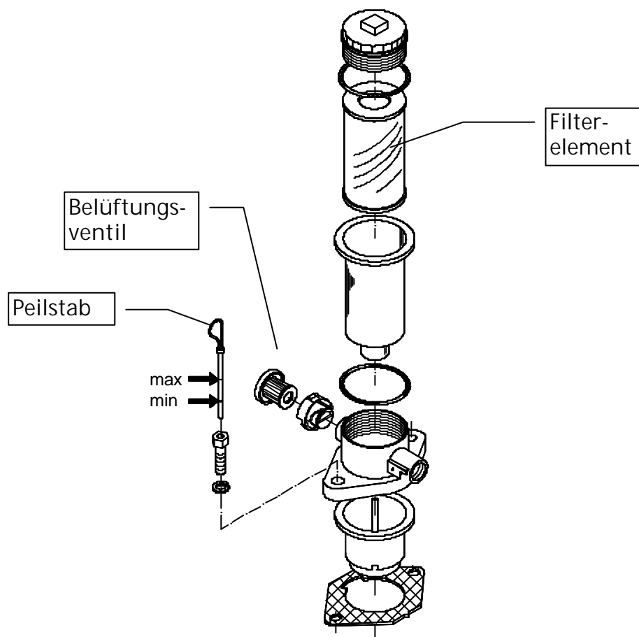
Rücklauffilter
