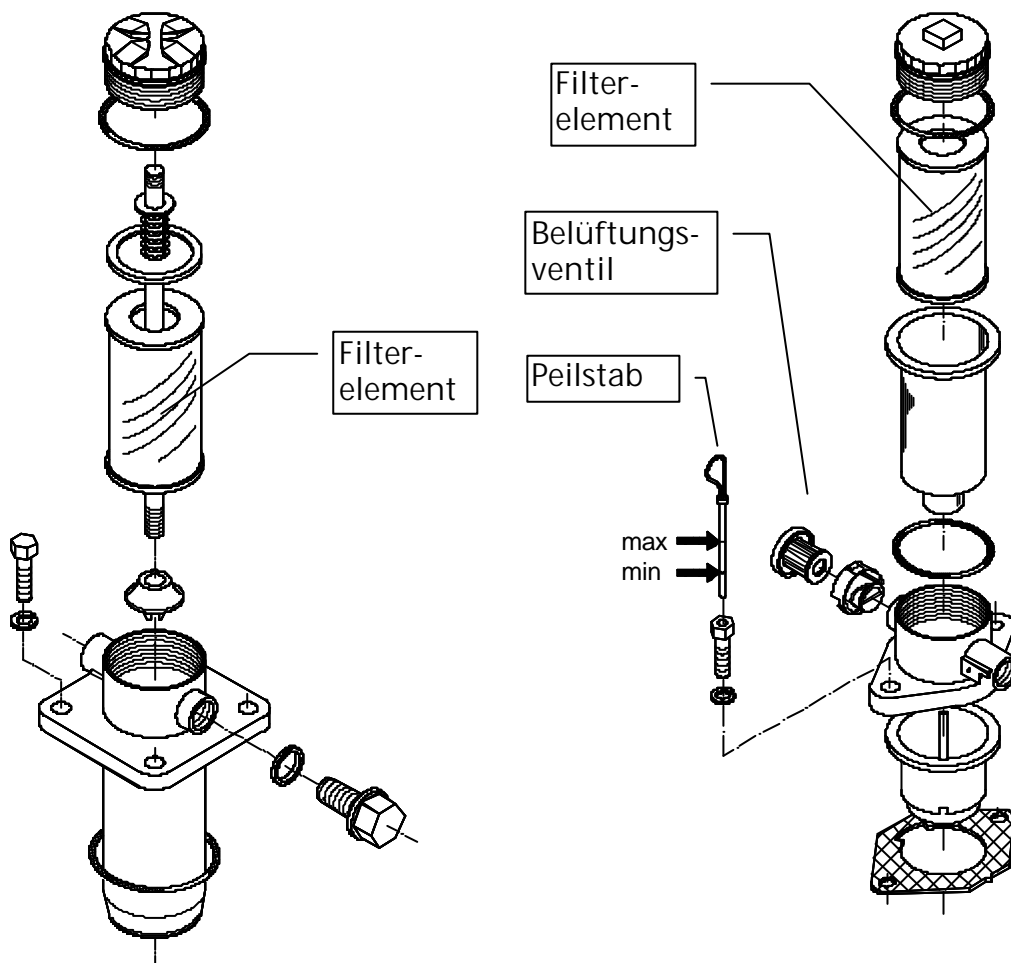
Saugfilter
