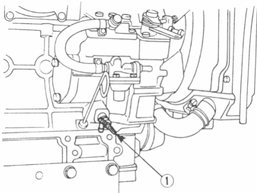
Hoflader 217S/ 221S/ 222S:
