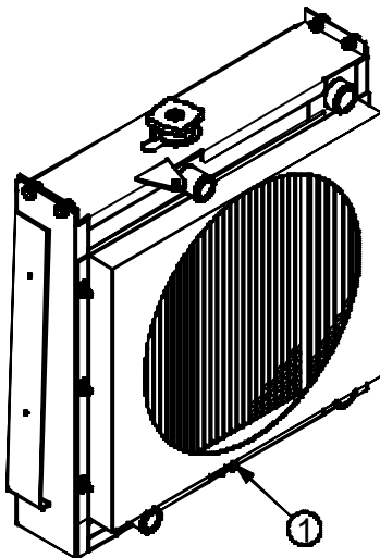
Hoflader 217S/ 221S/ 222S:
