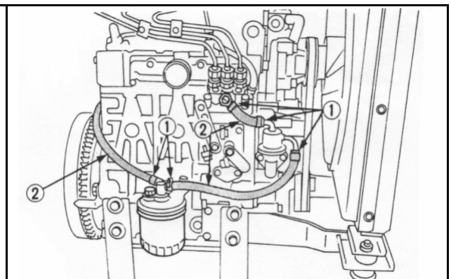
Lader 3036S/ 3045
