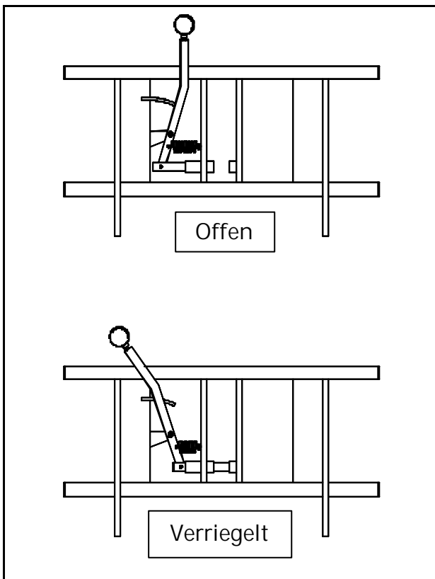
Abb. 2: Verriegeln des Arbeitswerkzeugs
