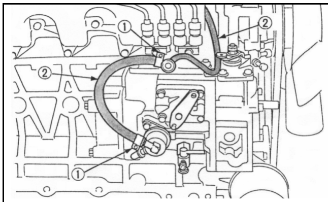
Lader 3036/ 4042/ 4048(S)
