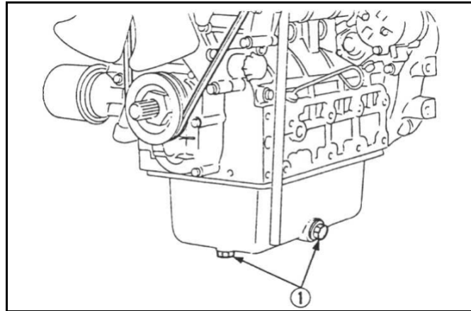
1) Ölablass-Schraube
