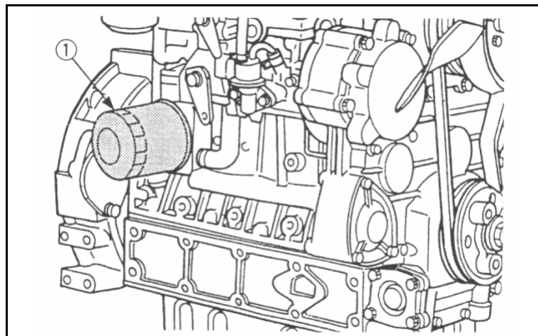
1) Ölfiltereinsatz
